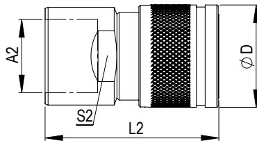
Engate Rápido Macho da Linha / Acople Rápido Macho de la Línea Superior / Male Quick Coupler Top Line
