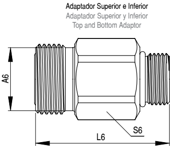
Adaptador Superior e Inferior / Adaptador Superior y Inferior / Top and Bottom Adaptor
