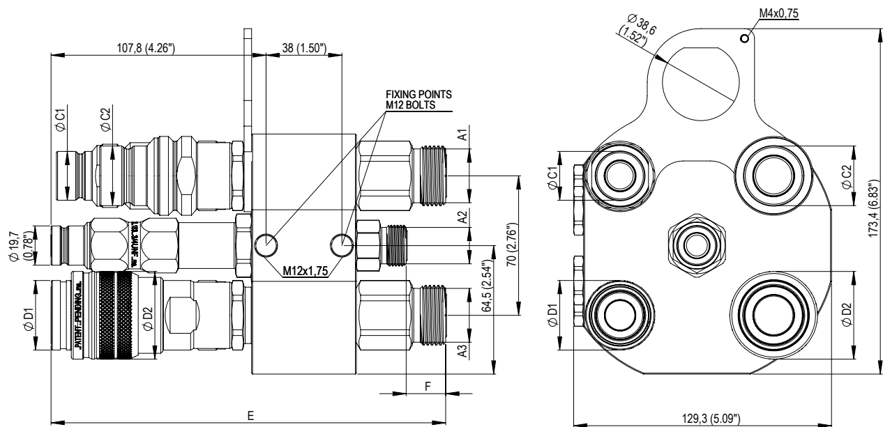
Bloco com Engates com Válvula de Despressurização / Bloque de Acoplamiento con Válvula de Despresurización / Decompression Block Coupler
