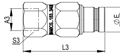
Engate Rápido Macho tamanho 9,5 (3/8") - DRAIN LINE Acople Rápido Macho tamanho 9,5 (3/8") - DRAIN LINE Male Quick Coupler size 9,5 (3/8") - DRAIN LINE
