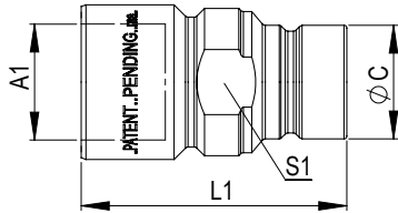
Engate Rápido Macho Tamanho 12,7 (1/2") ou 19,1 (3/4") Acople Rápido Macho Tamanho 12,7 (1/2") o 19,1 (3/4") Male Quick Coupler Size 12,7 (1/2") or 19,1 (3/4")
