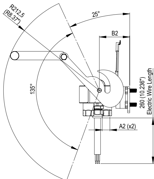
Parte Fixa / Parte Fija / Fixed Half
