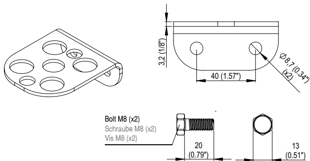
Docking for Mobile Half Stütze für den Beweglichen Teil Support pour la Partie Mobile
