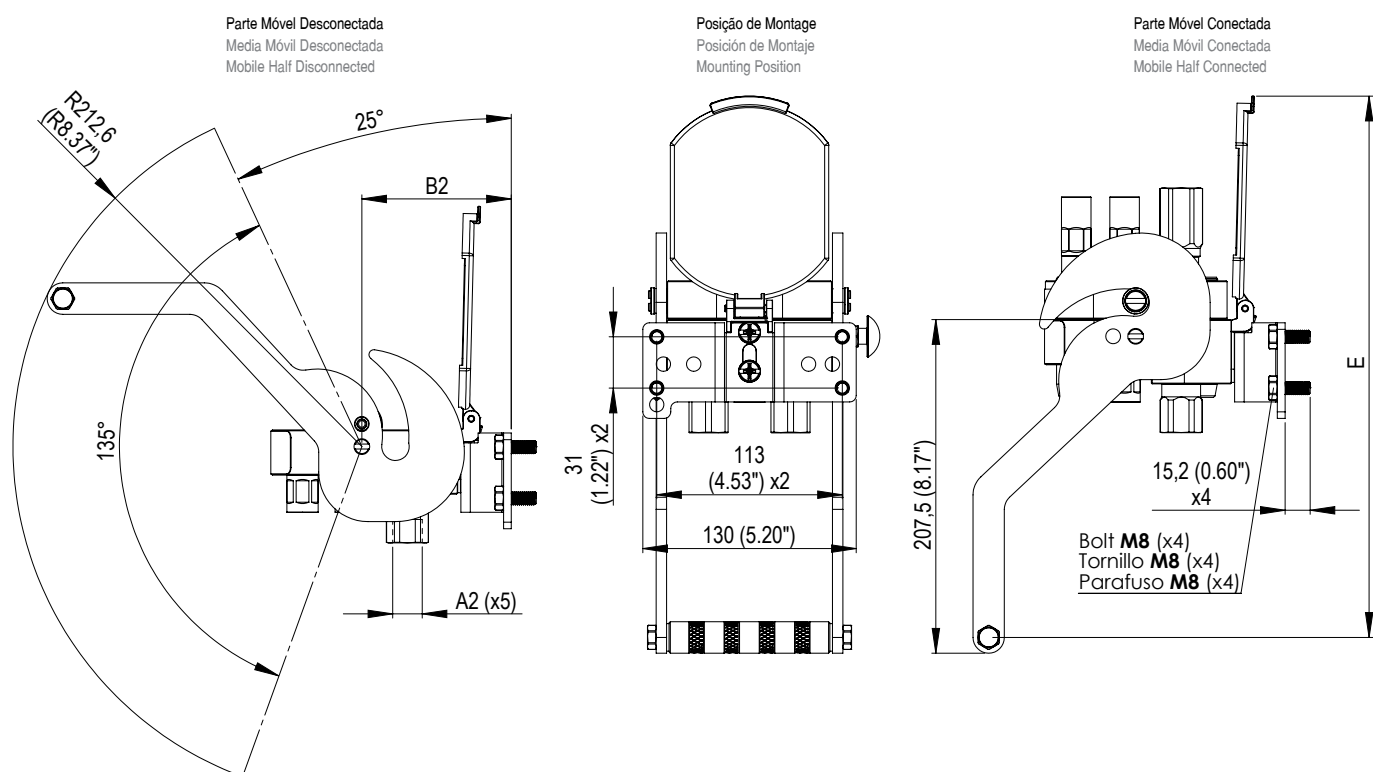
Parte Fixa / Parte Fija / Fixed Half
