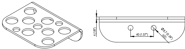
Apoio para Parte Móvel Soporte para Piezas Móviles Docking for Mobile Half
